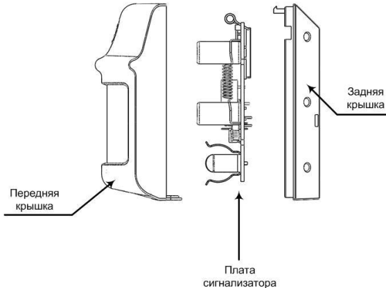
Рис.1 Конструкция сигнализатора
