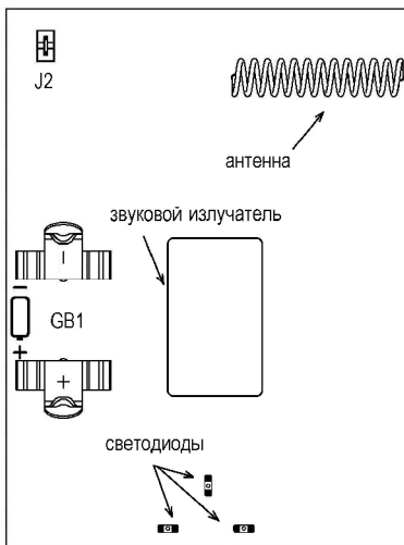
Рис. 2 Плата сирены
